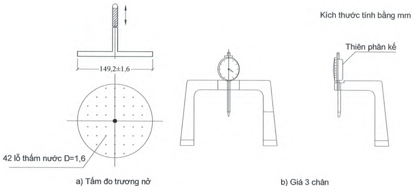
Hình 3 - Các dụng cụ đo độ trương nở
