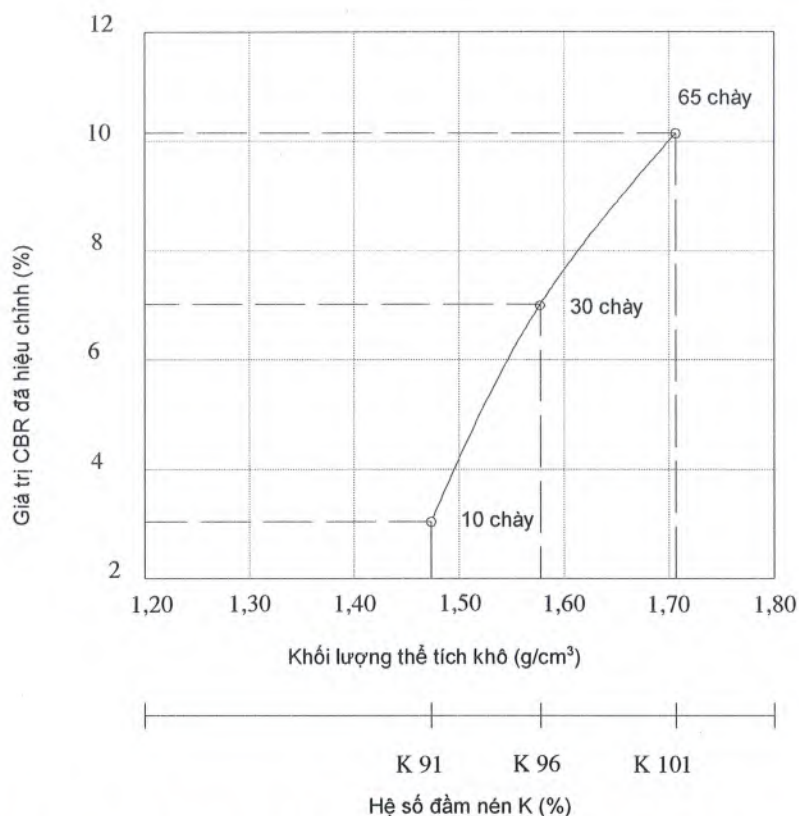
Hình 6 - Biểu đồ quan hệ CBR - Khối lượng thể tích khô
