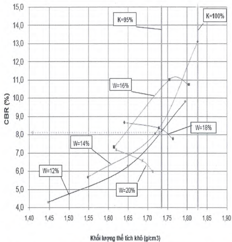
Hình B.3 – Quan hệ khối lượng thể tích khô – CBR theo các độ ẩm
