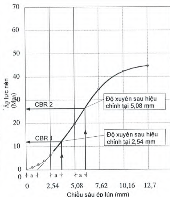
b) Hiệu chỉnh bằng cách dời gốc tọa độ
