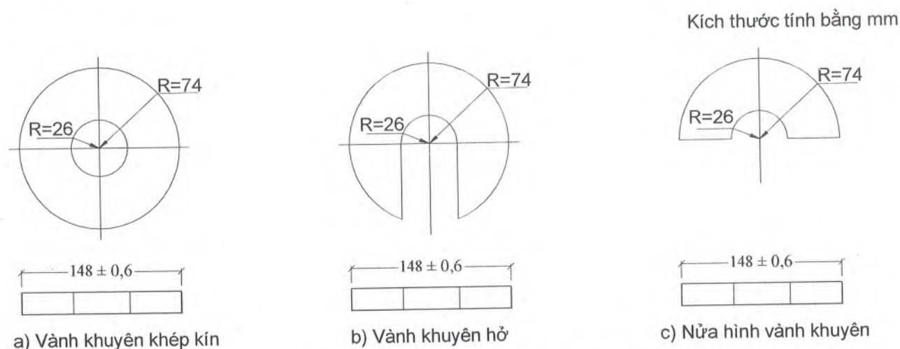
Hình 4 - Các vành khuyên tạo phụ tải
