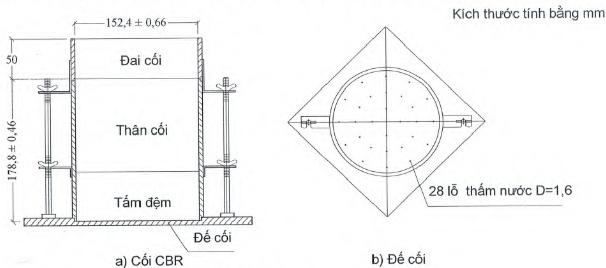
Hình 1 – Cối (khuôn) CBR
