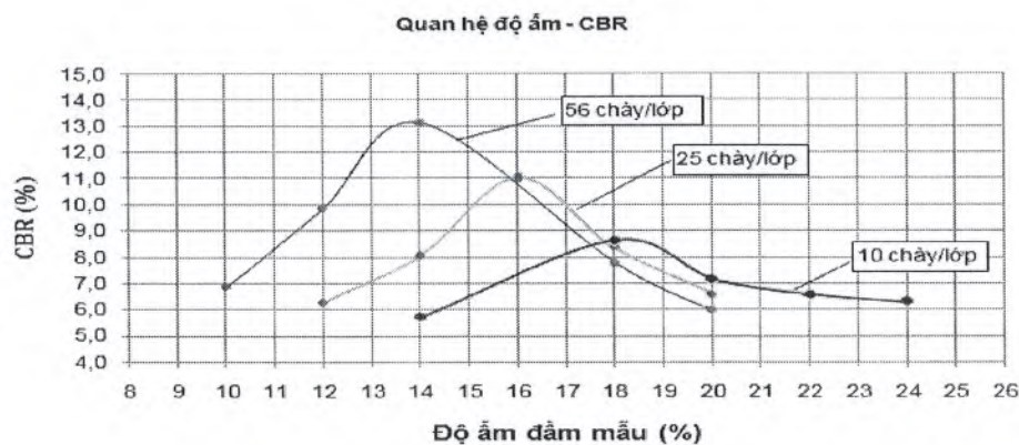
Hình B.2 - Quan hệ độ ẩm - CBR
