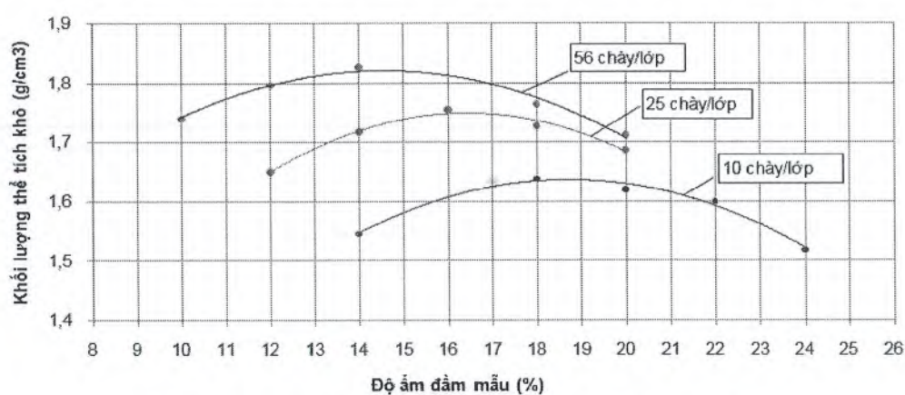
Hình B.1- Quan hệ độ ẩm - Khối lượng thể tích
